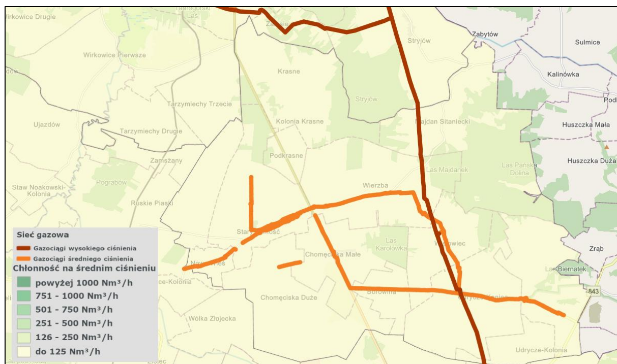
Rysunek 17. Przebieg infrastruktury gazowej średniego i wysokiego ciśnienia na terenie gminy Stary Zamość
